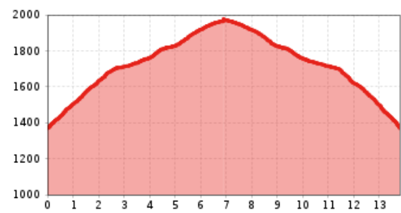
profilo altimetrico
